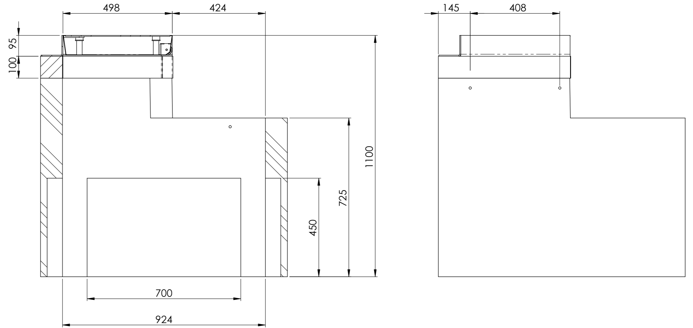
SCHNITT B-B
